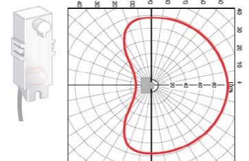
Sensor Arc Flash dan sensitifitasnya berdasarkan sudut
