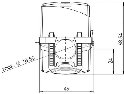
METSECT5CC...
